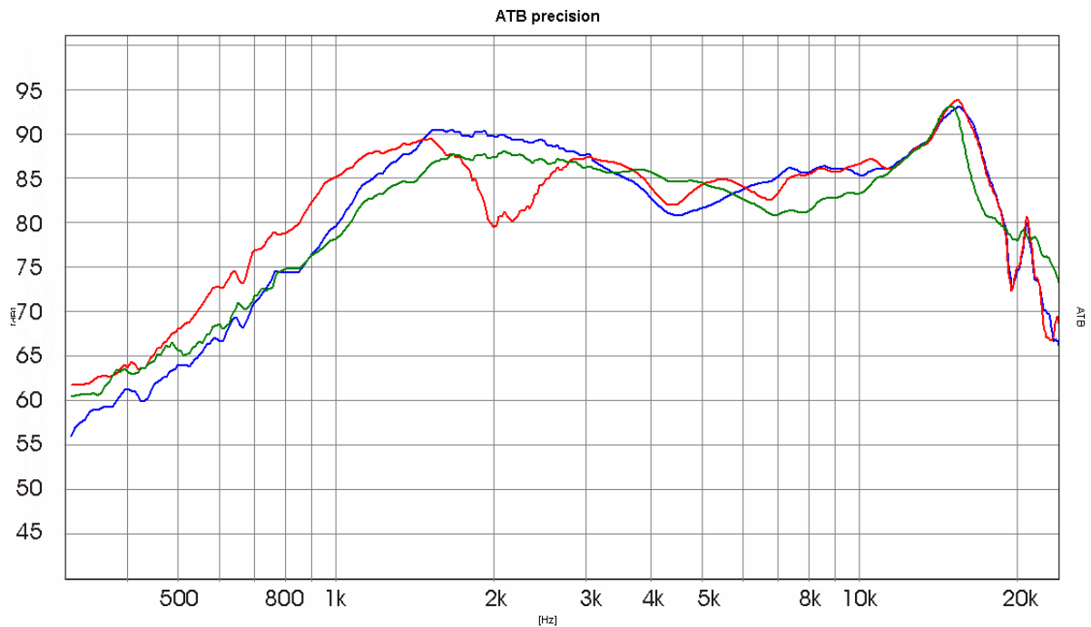
Bild 1.9 Frequenzgänge der Schallwände auf Achse gemessen Grün D = 8cm, blau D = 13cm, rot D = 27cm
