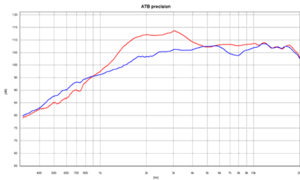
Bild 2.3 Vergleich der Frequenzgänge Die blaue Kurve zeigt den Frequenzgang der Kalotte und die rote den des Waveguides auf der Achse gemessen. Für die tieferen Frequenzen wird der Schalldruck durch den Strahlungswiderstand des Waveguides erhöht.
