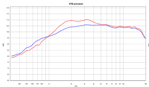
Bild 2.4 Schallleistung Die blaue Kurve zeigt die Schallleistung über die Frequenz der Kalotte und die rote die des Waveguides.
