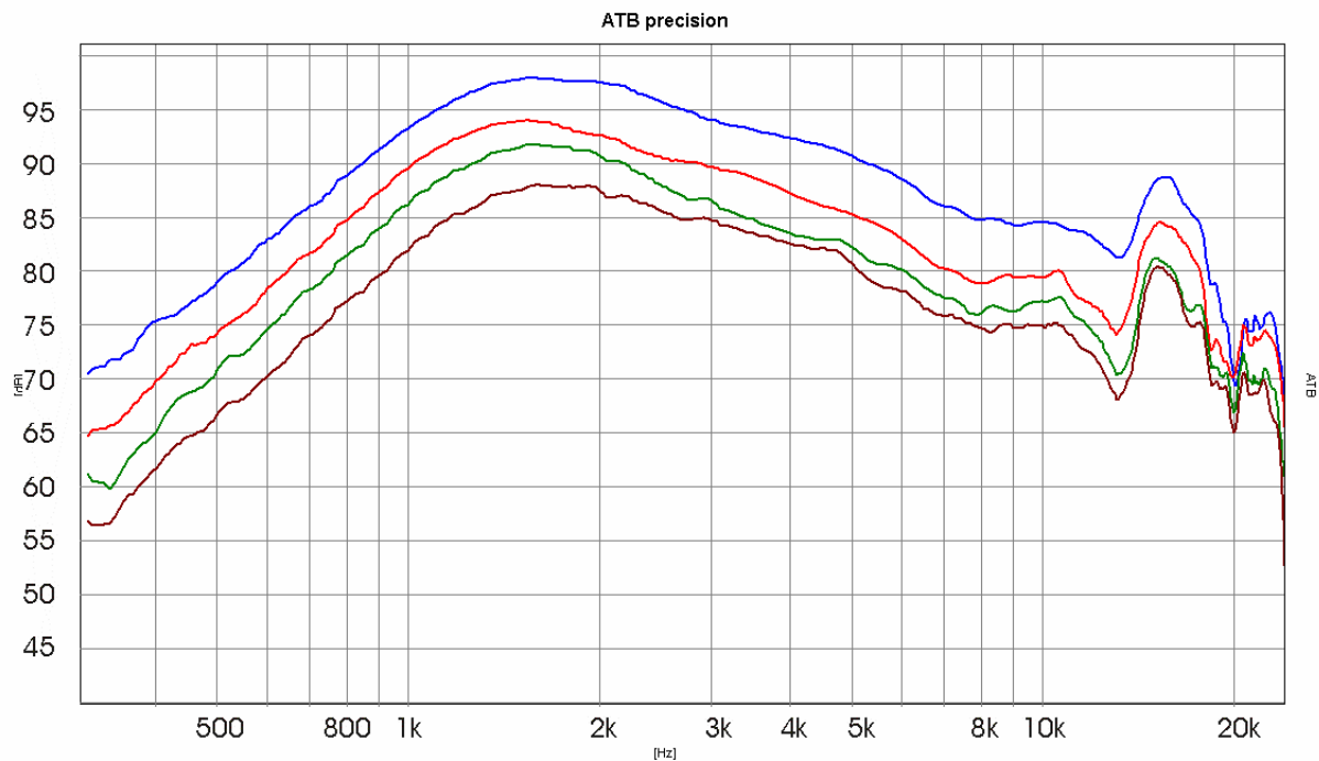
Bild 1.13 Frequenzgänge in verschiedenen Abständen auf der Schallwand gemessen Abstand vom Mittelpunkt: blau = 4,5cm, rot = 7,5cm, grün = 10,5cm, braun = 13,5cm
