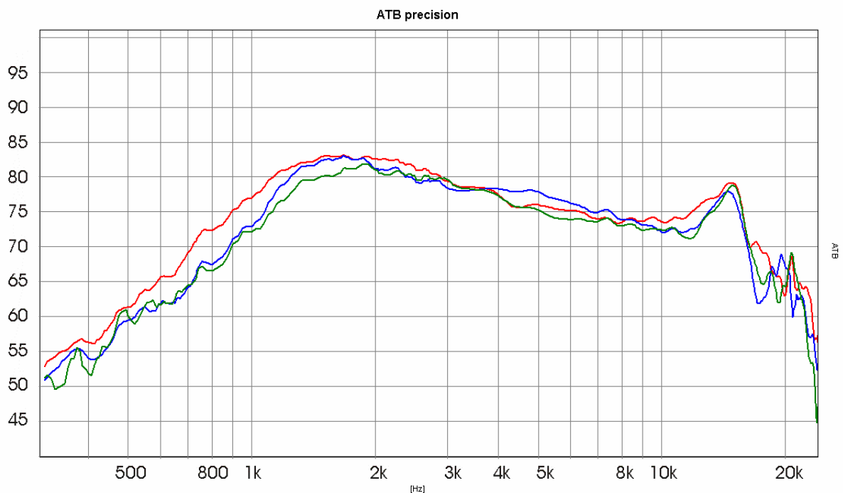
Bild 1.10 Frequenzgänge der Schallwände unter 45° gemessen Grün D = 8cm, blau D = 13cm, rot D = 27cm
