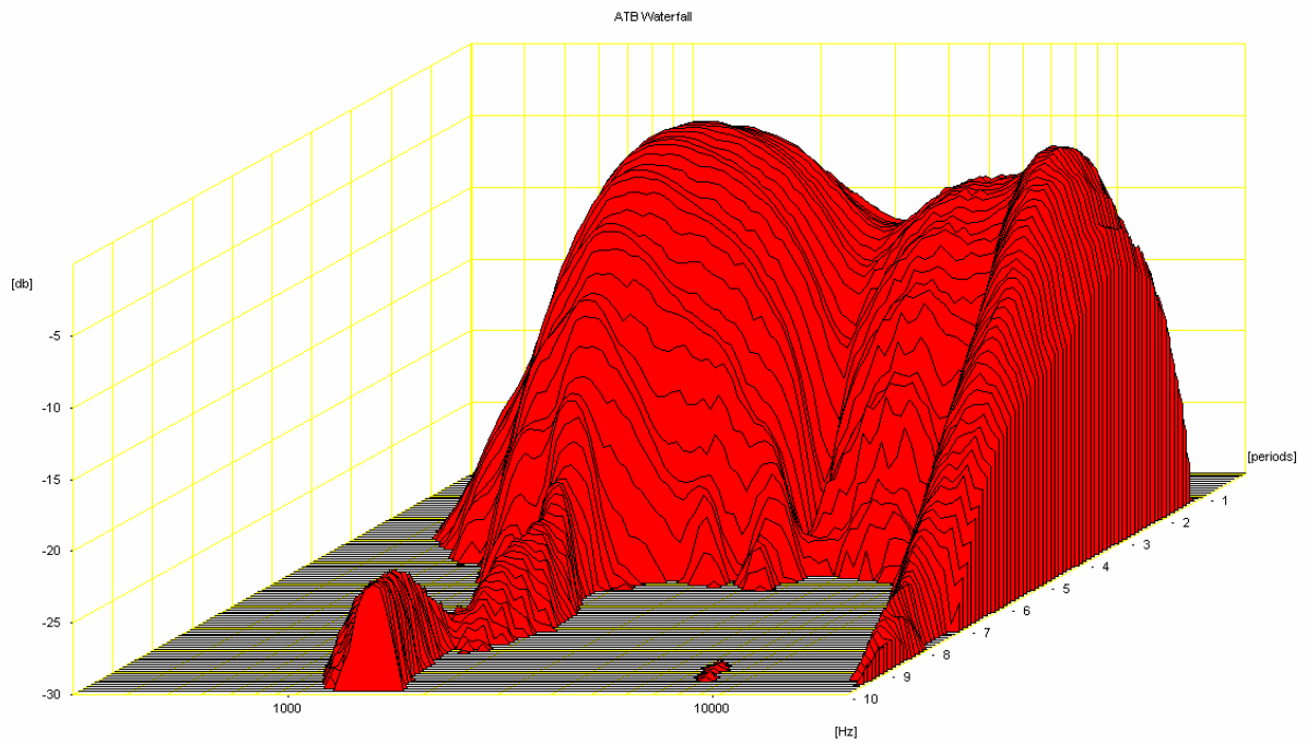
Bild 1.11 Wasserfalldiagramm
