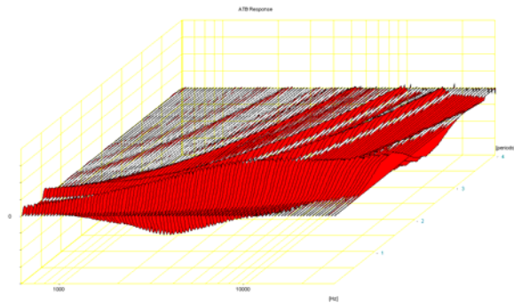
Bild 2.8 Impulsverhalten Kalotte
