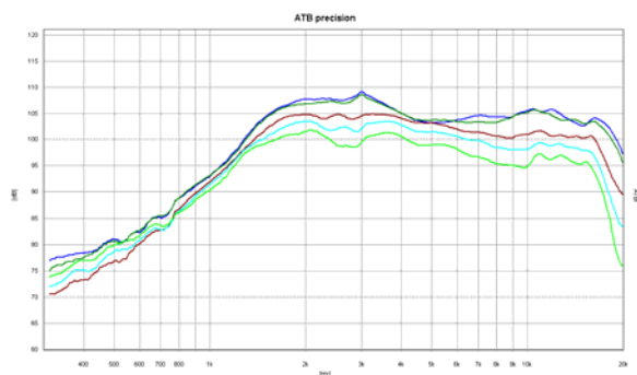
Bild 2.6 Abstrahlverhalten Waveguide Blau =0°, dunkelgrün =15°, rot =30°, hellblau =45°, hellgrün = 60°. Mit größerem Winkel wird der Schalldruck geringer, die Charakteristik der Kurve bleibt. Dies zeigt, dass der Klang für verschiedene Sitzpositionen gleich bleibt.
