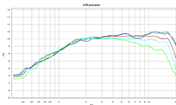
Bild 2.5 Abstrahlverhalten Kalotte Blau =0°, dunkelgrün =15°, rot =30°, hellblau =45°, hellgrün = 60°. Mit größerem Winkel fällt die Kurve zu höheren Frequenzen ab. Hierdurch wird der Klang von der Sitzposition abhängig. Mit größerem Winkel besteht ein Höhenabfall.
