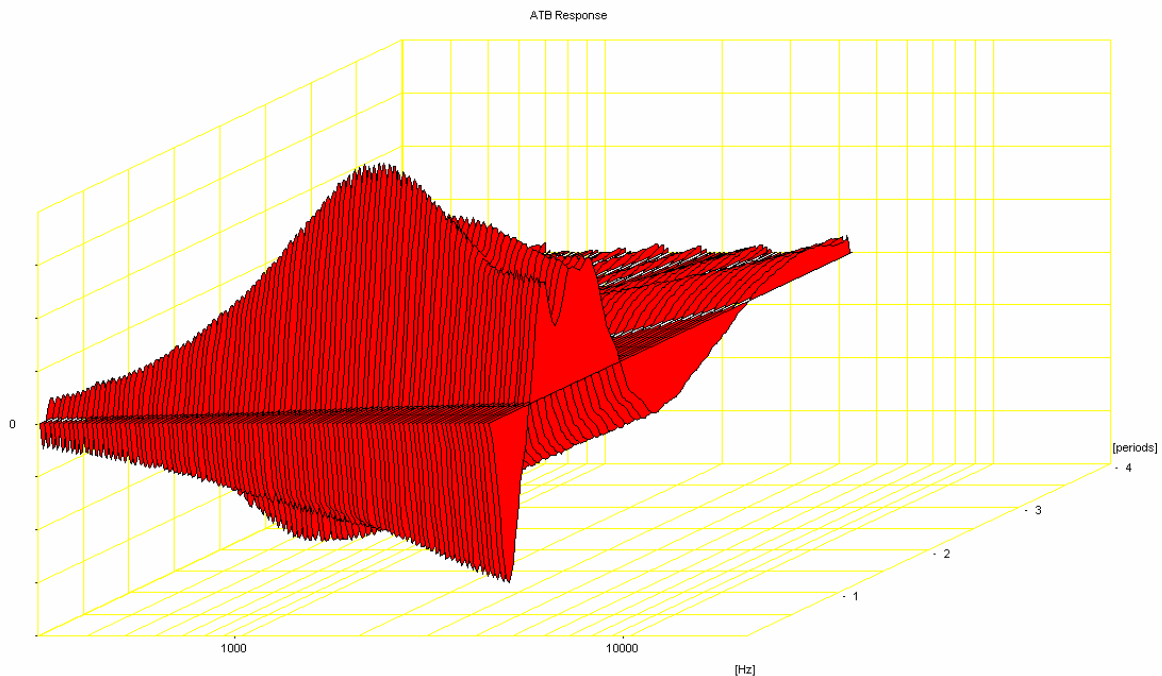
Bild 1.14 Dynamic-Measurement Messung bei der Schallwand D = 8
