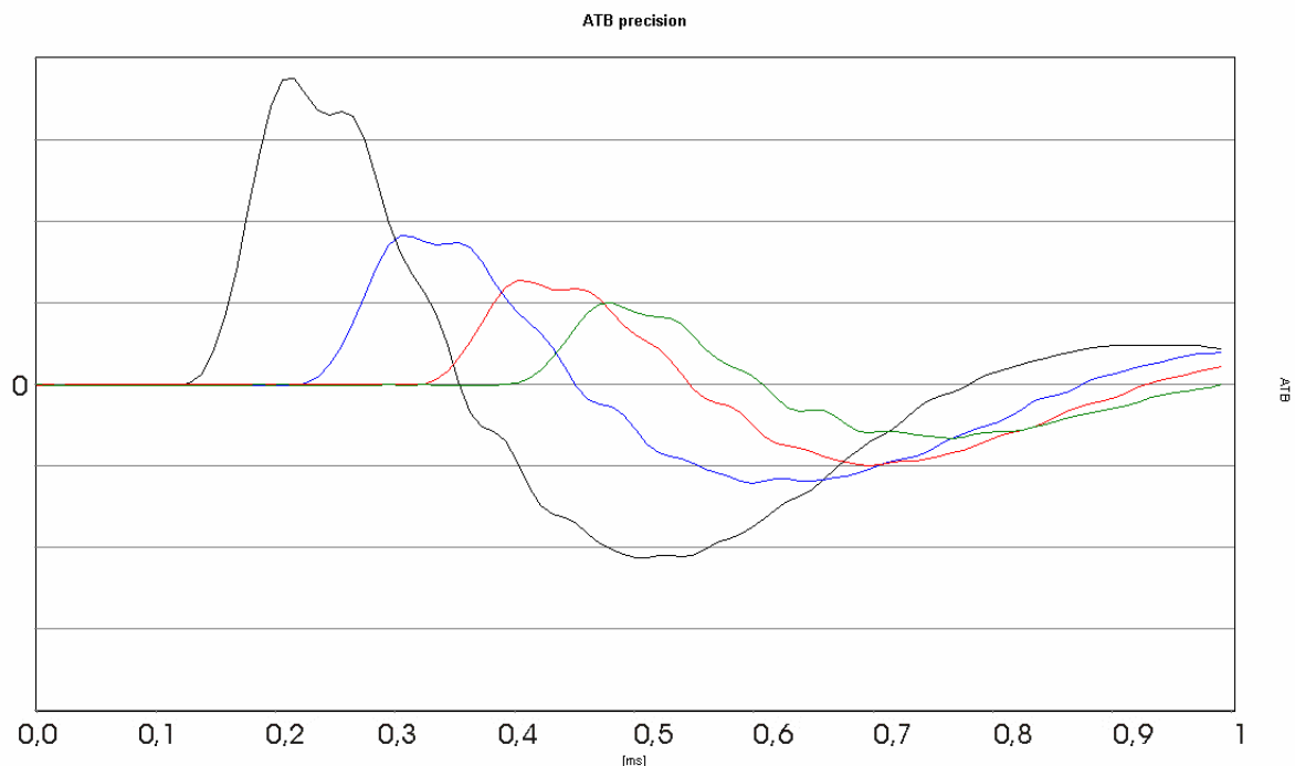
Bild 1.12 Sprungantwortmessungen auf der Schallwand
