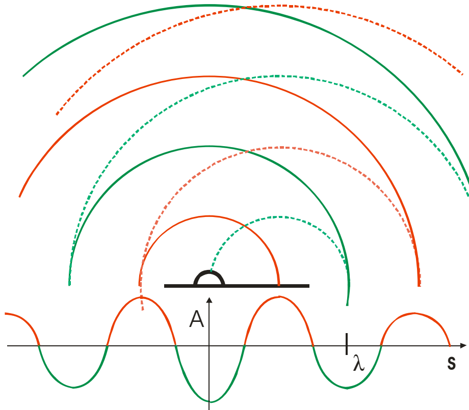
Bild 1.1 Schallfeld
