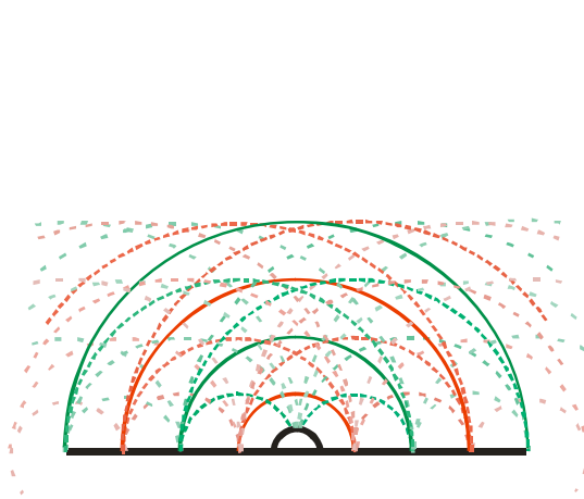
Bild 1.2 \lambda < D
