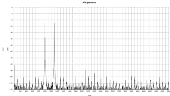
Das Frequenzspektrum des Signals 13
