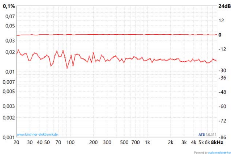
Klirrfaktor THD
