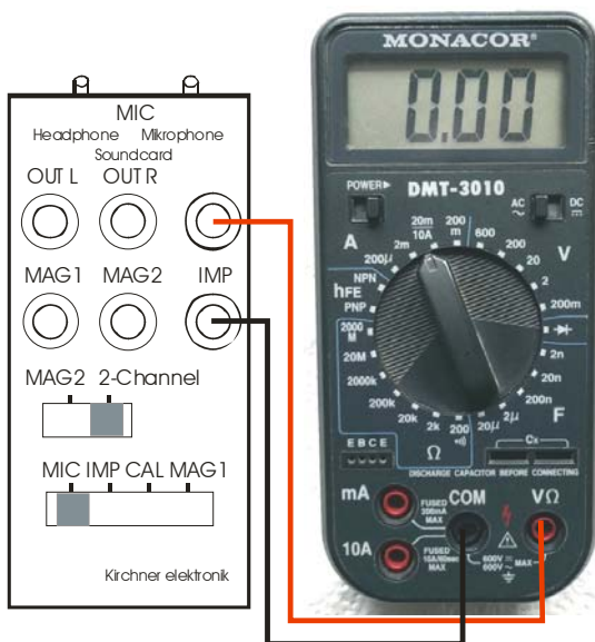
Messaufbau mit dem ATB Audio Analyzer Test-Adapter
