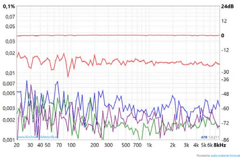
Klirrfaktor THD
