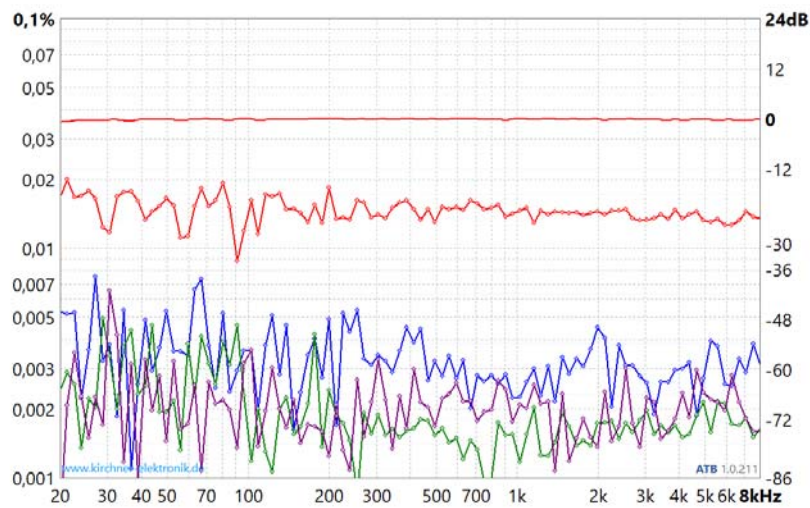
Klirrfaktor THD
